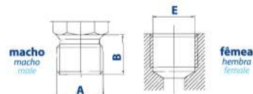
Cônica Cônica Flare Rosca BSP Rosca BSP Thread BSP
